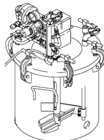
236154 - 72 L - 7 bar avec agitateur 0,4 Kw - réducteur 20:1 - pales diam 216 mm
